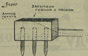
Вот как устроен ящик — устой плотины.
