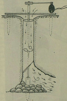
Схема самой простой самодельной турбины.
