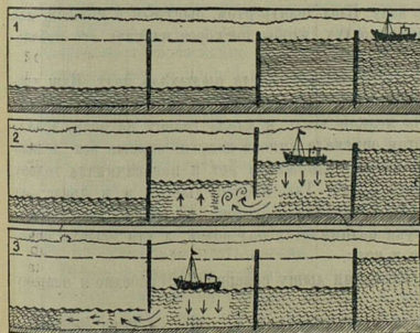
Схема шлюза.
